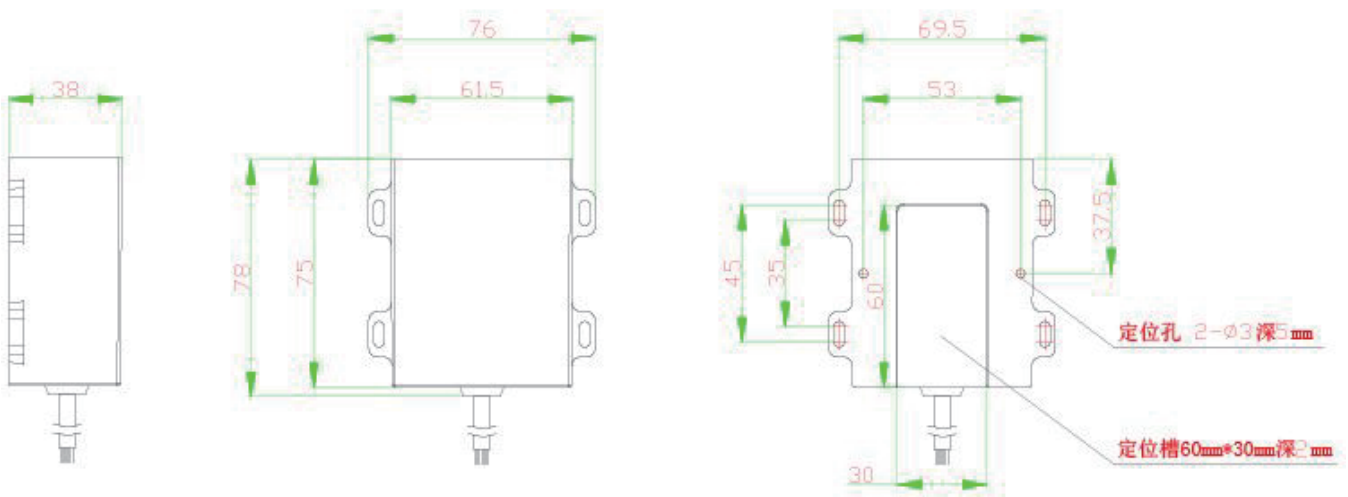
左視圖
